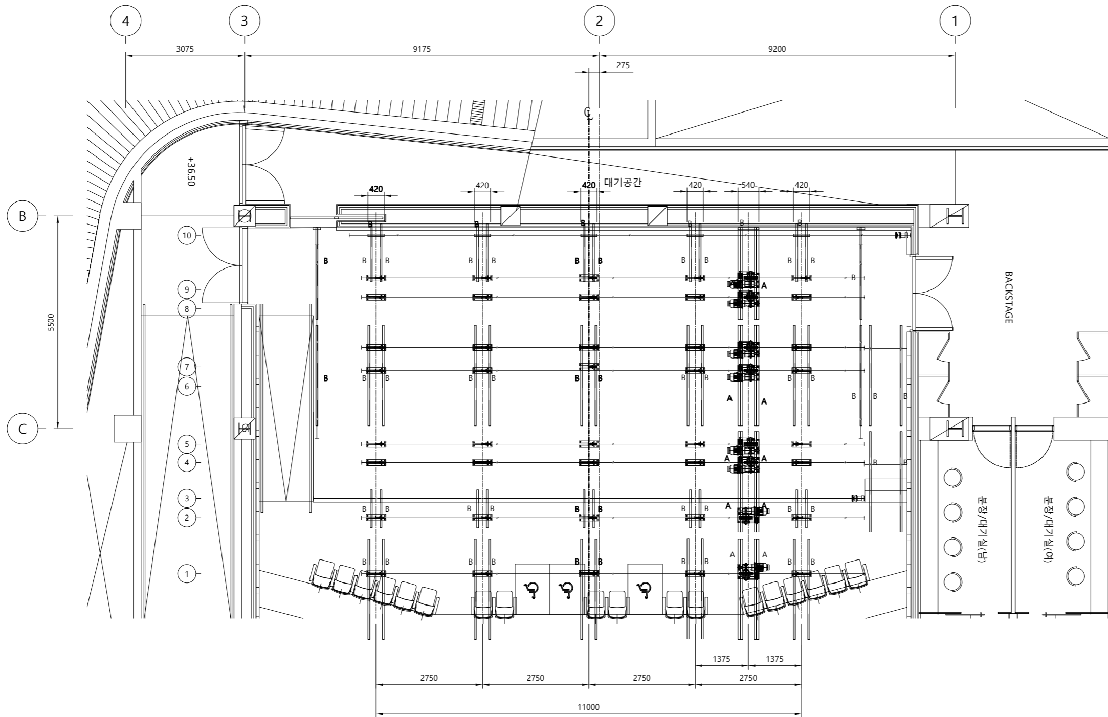
1 공연장 무대조명 설비 평면도-3 SCALE : 1 / 100
