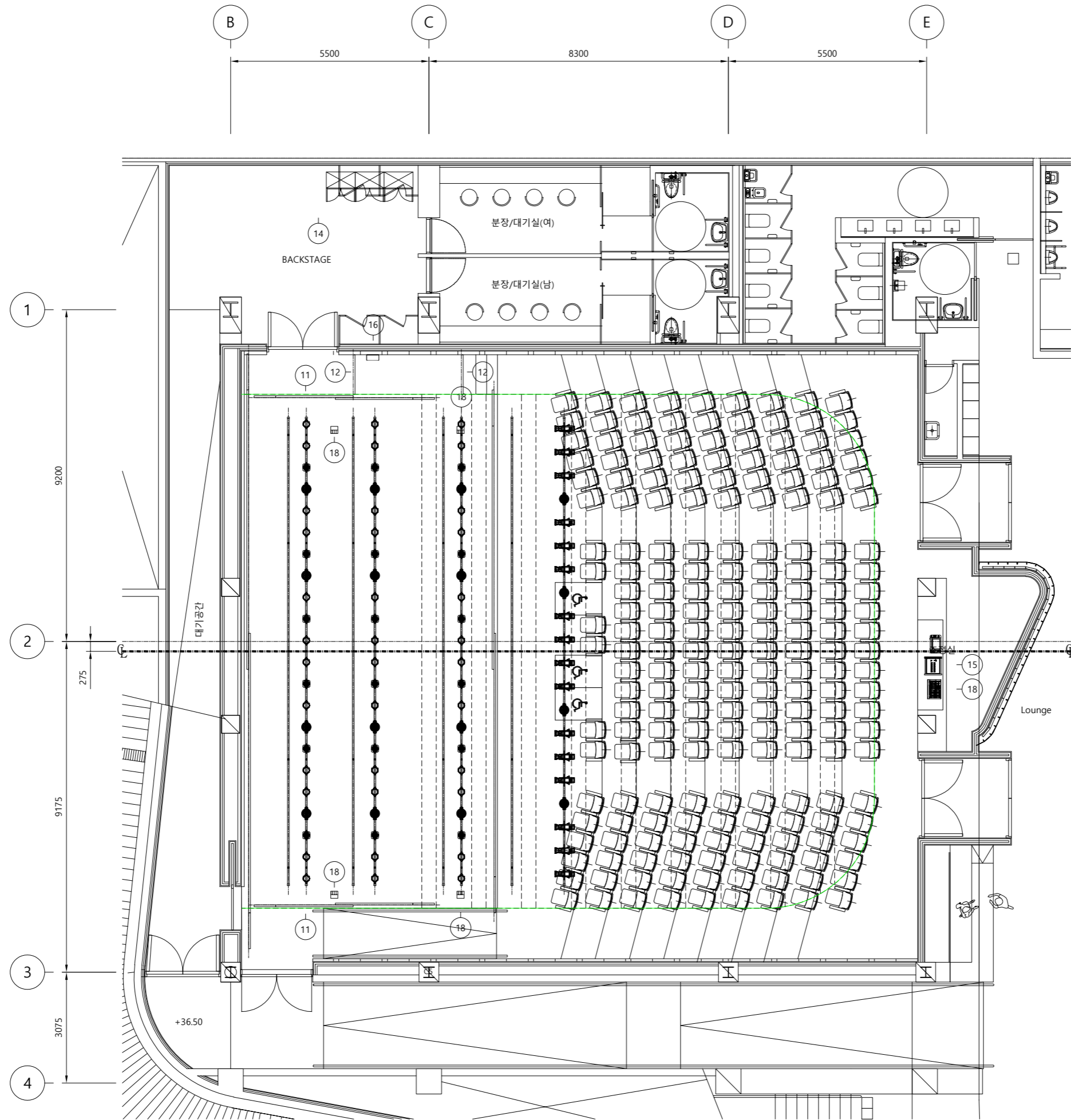
1 공연장 무대조명 설비 평면도-1 SCALE : 1 / 120
